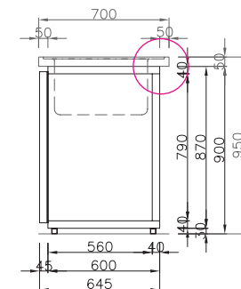
Schnitt links: Abdeckung mit um- laufendem Wulstrand
