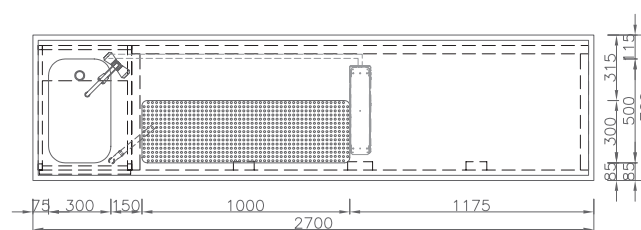
Gläserdusche in Siebplatte eingebaut
