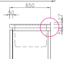
Schnitt links: Abdeckung mit um- laufendem Wulstrand
