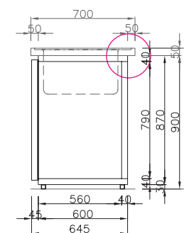
Schnitt links: Abdeckung mit um- laufendem Wulstrand
