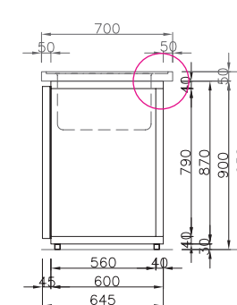
Schnitt links: Abdeckung mit um- laufendem Wulstrand
