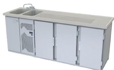
Modell N3/2L B 2.450 x T 650/700 x H 950 mm Modell N3/2R spiegelbildlich mit Becken rechts
