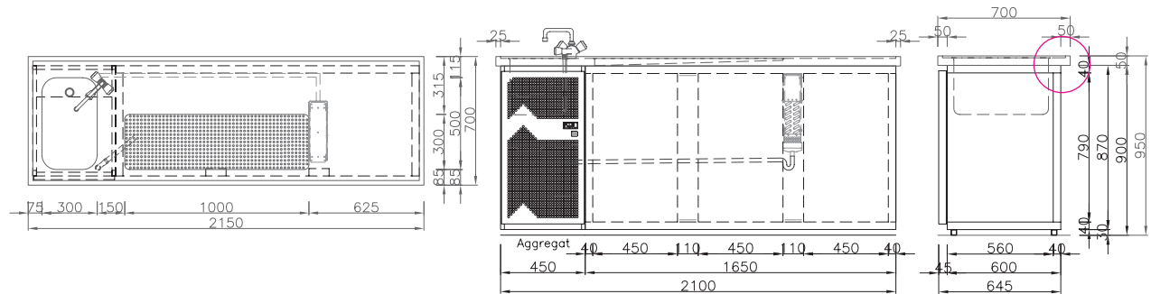
Gläserdusche in Siebplatte eingebaut
