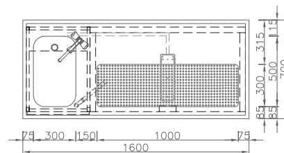
Gläserdusche in Siebplatte eingebaut
