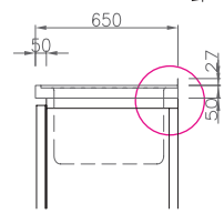
Schnitt links: Abdeckung mit um- laufendem Wulstrand
