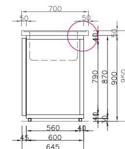
Schnitt links: Abdeckung mit um- laufendem Wulstrand
