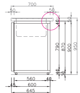
Bohrung für Schanksäule
