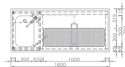
Gläserdusche in Siebplatte eingebaut
