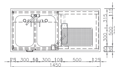
Gläserdusche in Siebplatte eingebaut
