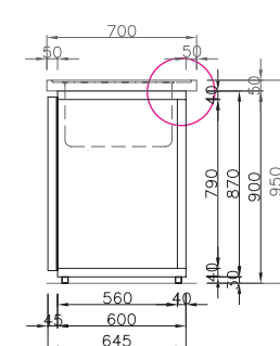
Schnitt links: Abdeckung mit um- laufendem Wulstrand Schnitt rechts: Abdeckung mit gast- seitiger Hochkantung
