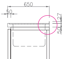
Schnitt rechts oben: Abdeckung mit um- laufendem Wulstrand
