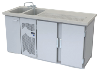
Modell A2/2L B 1.900 x T 650/700 x H 950 mm Modell A2/2R spiegelbildlich mit Becken rechts
