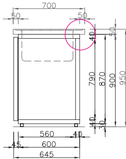
Fassrutsch- leisten
