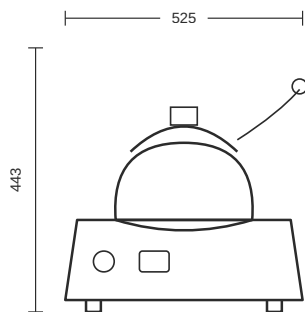
Frontansicht · Breite und Höhe in mm
